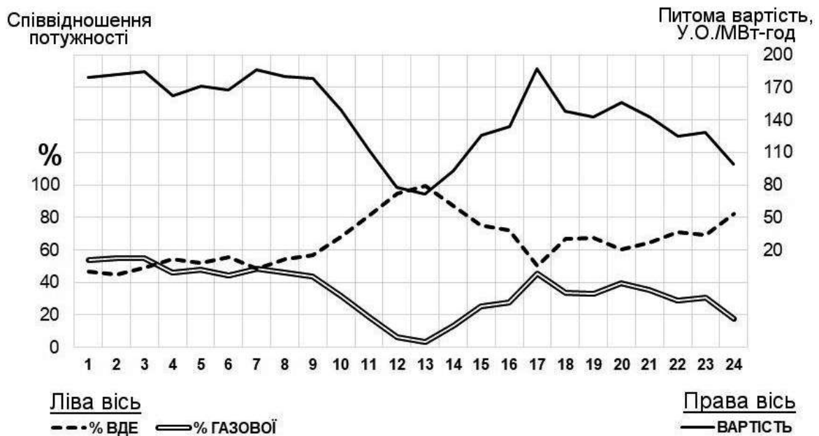
Рис. 2. Залежність питомої вартості теплопостачання від співвідношення потужності ВДЕ та газової генерації
